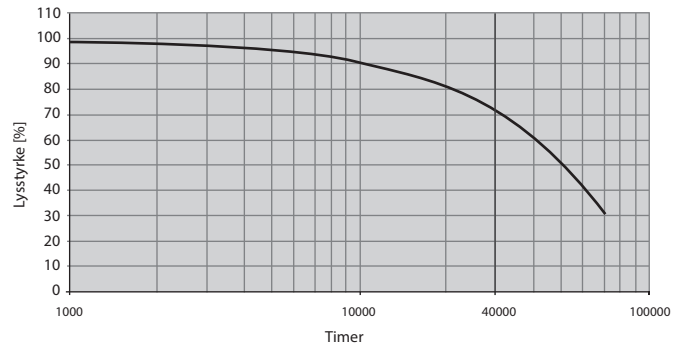
Diagram 1: Beregnet lysstyrke over tid
