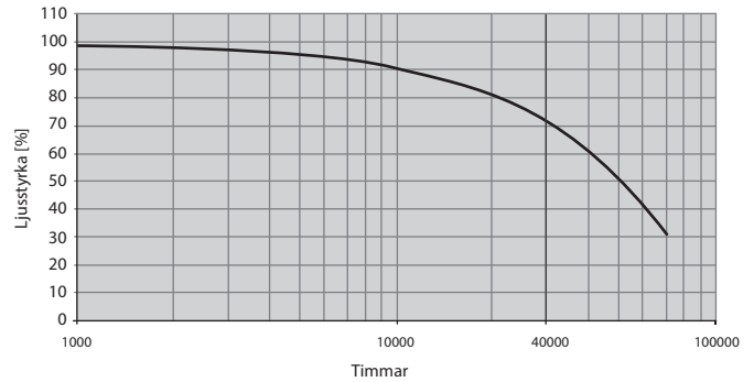
Diagram 1: Beräknad ljusstyrka över tid
